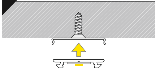
držák U5 otvor zahloubený cone U5 mounting plate
